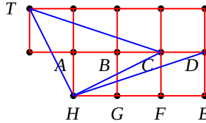
Figura A.4: Problema 584.
