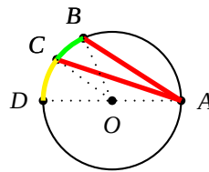
Figura 7.30: Teorema 566. Caso III.
