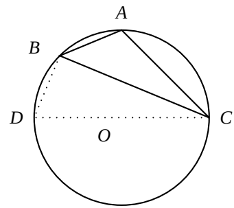
Figura 7.183: Generalización de la ley de los senos. \hat{A} obtuso.
