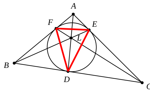
Figura 7.185: Punto de Gergonne y triángulo de Gergonne.
