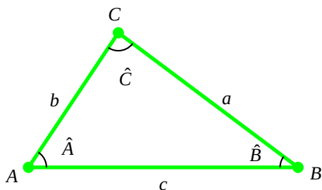
Figura 7.127: Notación para triángulos.
