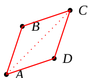
Figura 7.19: Cuadrilátero simple y convexo.
