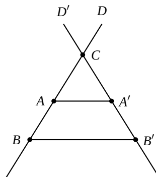
Figura 7.154: Corolario del teorema de Thales
