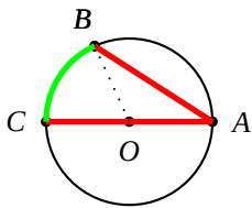
Figura 7.28: Teorema 566. Caso I.
