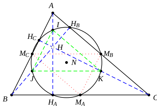
Figura 7.187: Círculo de nueve puntos de Euler-Feuerbach.
