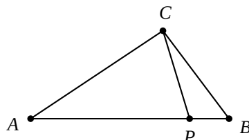
Figura 7.133: Teorema de la bisectriz angular.
