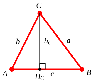
Figura 7.129: Fórmulas de área.
