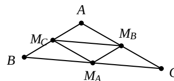
Figura 7.181: El triángulo medial.
