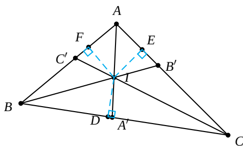
Figura 7.184: El incentro. Teorema 876.
