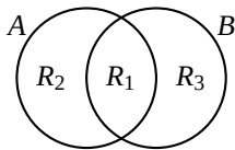
Figura 3.5: Inclusión-exclusión para dos conjuntos.
