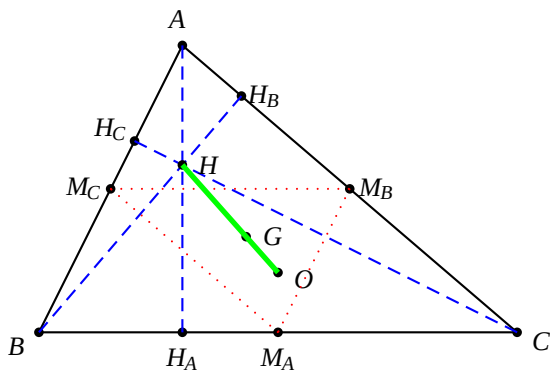
Figura 7.186: Recta de Euler.
