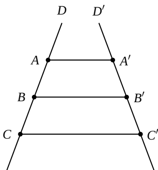
Figura 7.153: Teorema de Thales.
