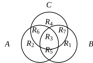
Figura 3.6: Inclusión-exclusión para tres conjuntos.
