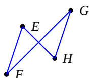
Figura 7.20: Cuadrilátero no simple.
