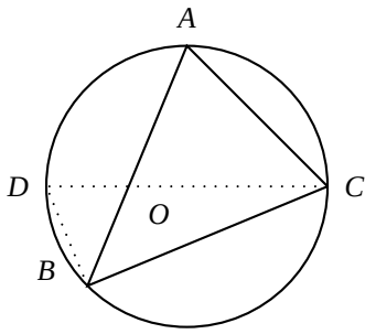
Figura 7.182: Generalización de la ley de los senos. \hat{A} agudo.
