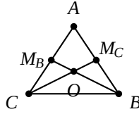
Figura A.6: Problema 639.
