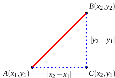
Figura 7.139: Distancia entre dos puntos.
