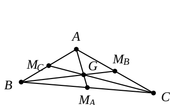
Figura 7.179: El baricentro. Teorema 862.
