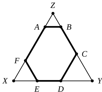
Figura A.5: Problema 594.
