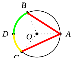
Figura 7.29: Teorema 566. Caso II.
