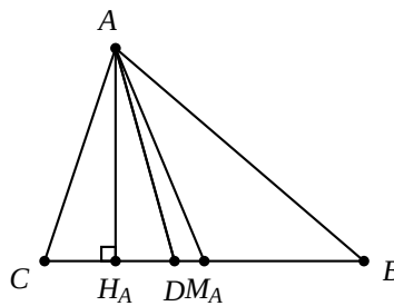
Figura A.7: Problema 691.
