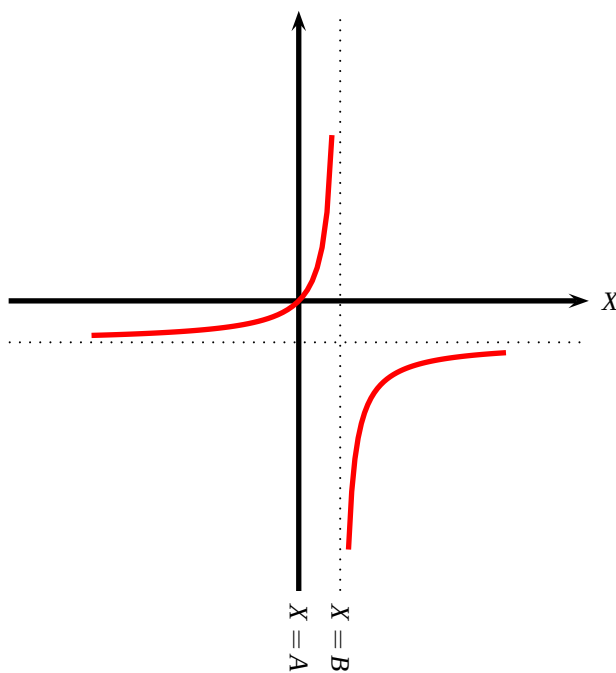
Figura 7.152: Razón \frac{\overline{AX}}{\overline{XB}} (eje vertical) contra X (eje horizontal).
